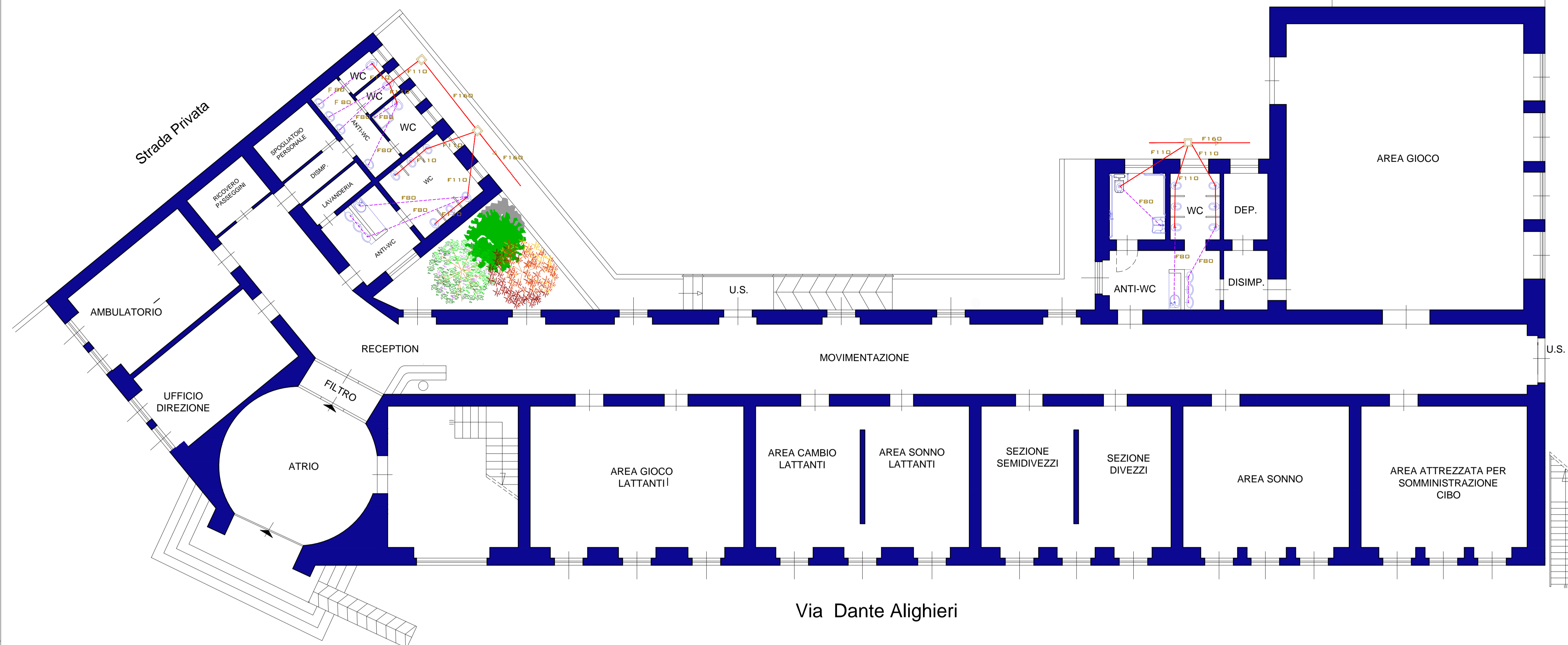
PIANTA RETE FOGNANTE SCALA 1:100
