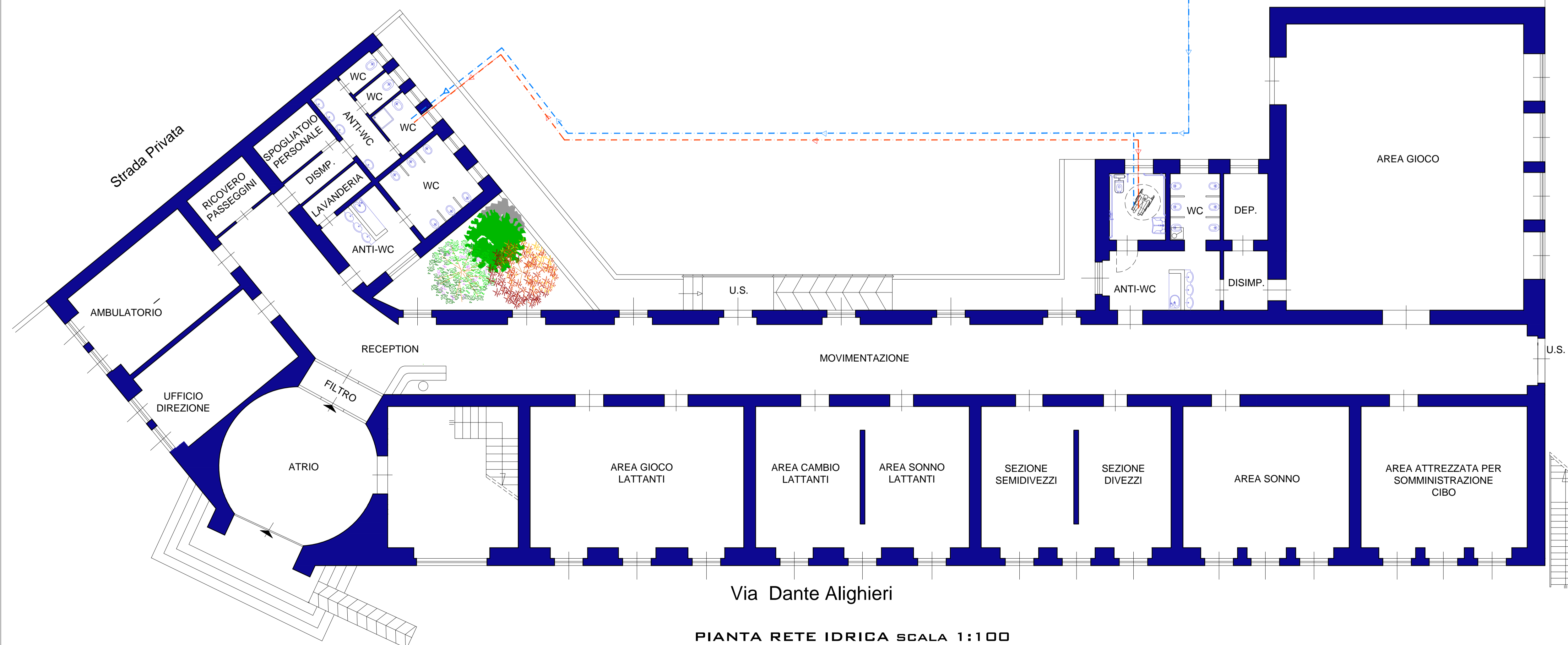
PIANTA RETE IDRICA SCALA 1:100
